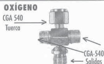
CGA-540 PIEZA NO. C-4540
